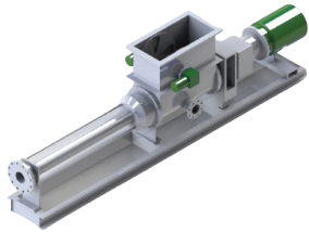
피스톤 펌프
